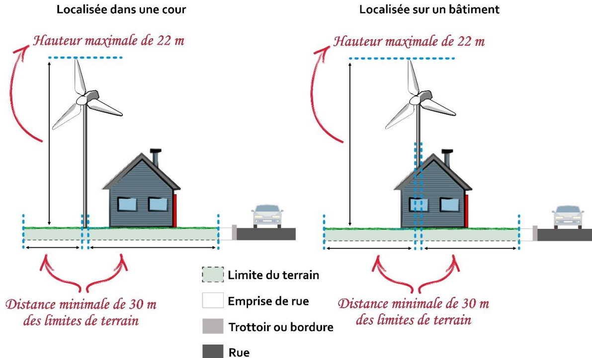
Figure 53 : Dimensions et implantation d'une éolienne domestique
