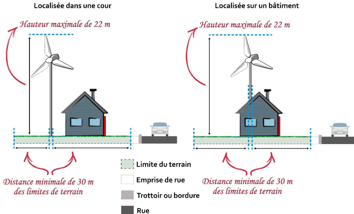
Figure 82 : Dimensions et implantation d'une éolienne domestique
