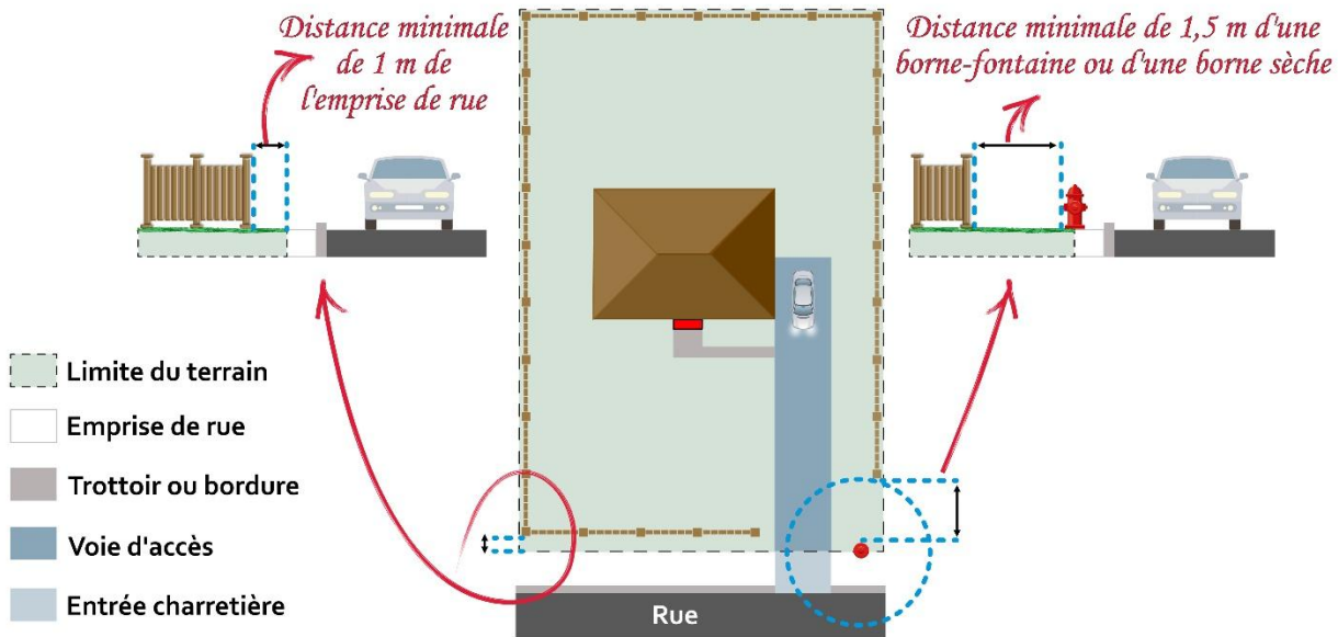
Figure 50 : Implantation d'une clôture
