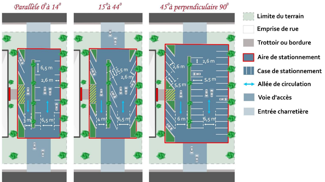
Figure 39 : Dimensions d'une case de stationnement
